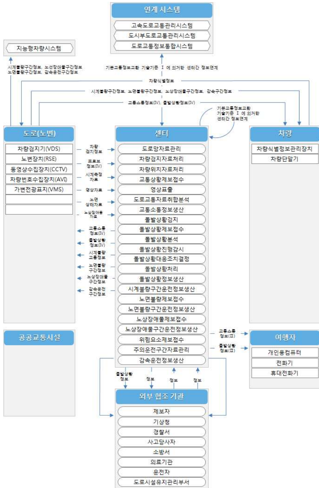
[그림 7-5] ATMS 단위시스템과 물리적 구성요소들 간 자료 흐름도
