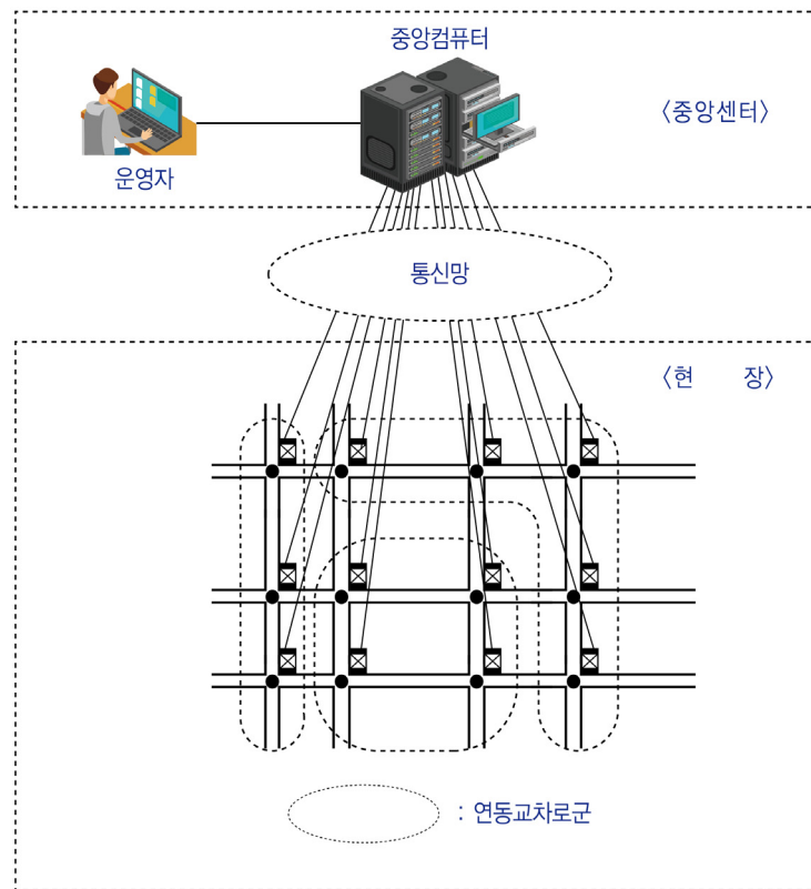
그림 1-6 센터 컴퓨터에 의한 중앙연동방식
